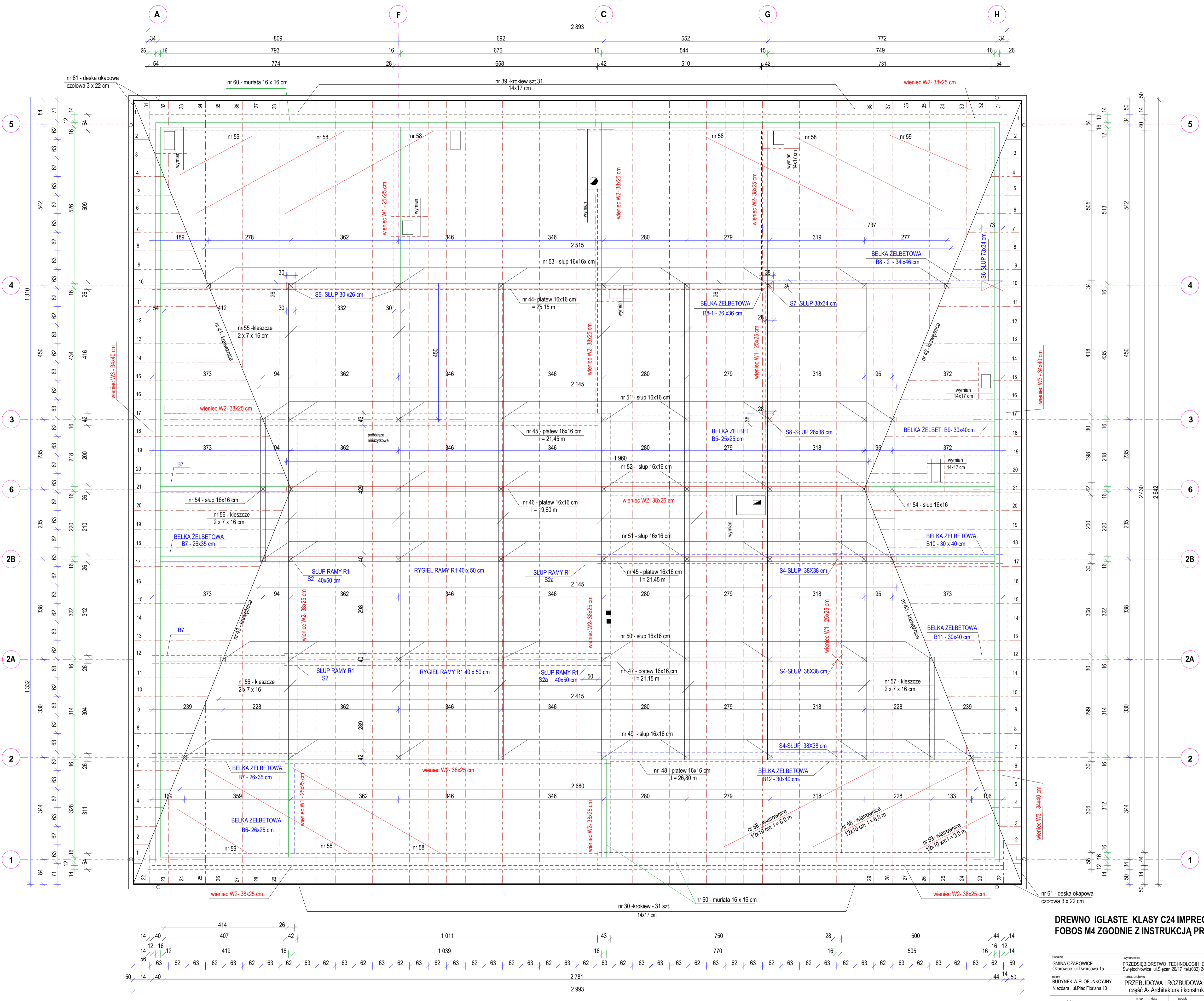
RZUT KONSTRUKCJI DACHU skala 1 : 50
