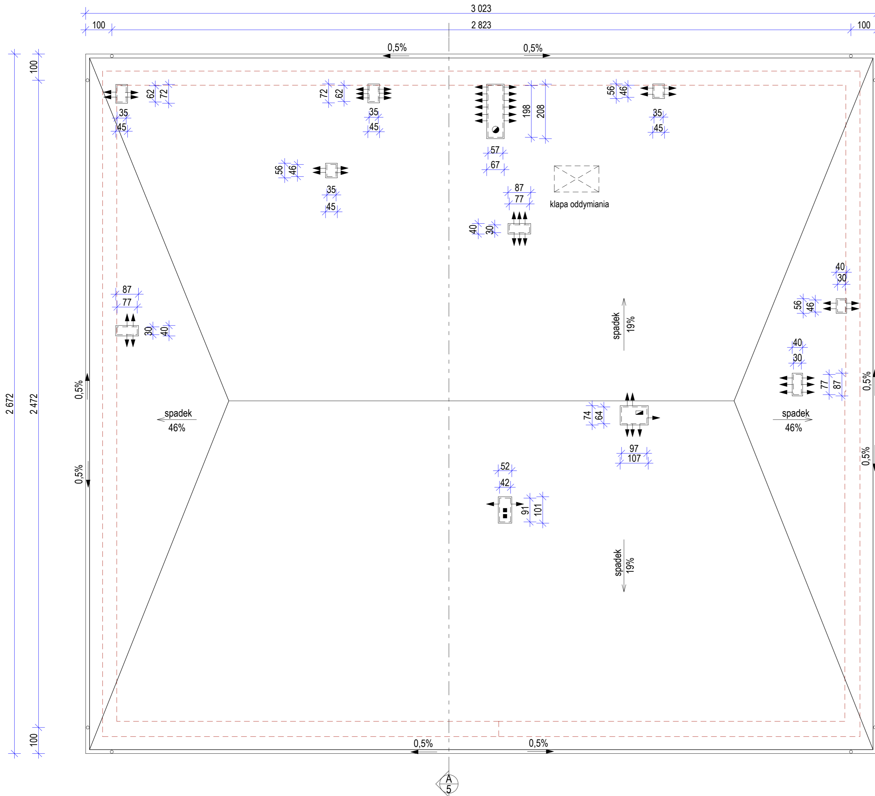
RZUT DACHU skala 1 : 100
