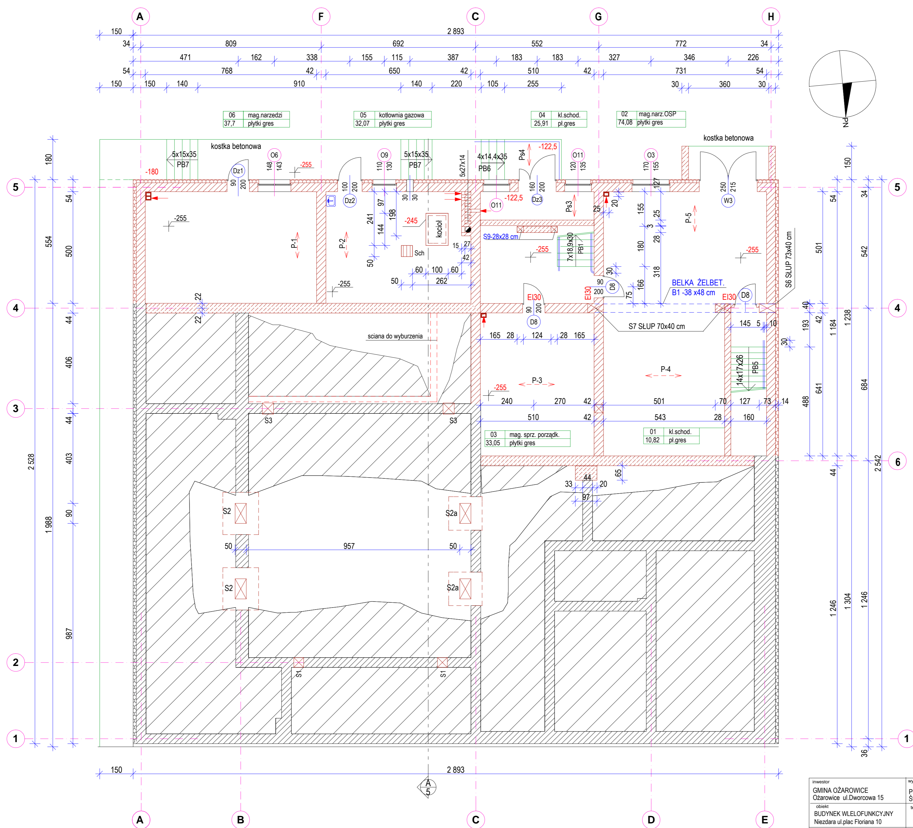
RZUT PIWNIC skala 1:100
